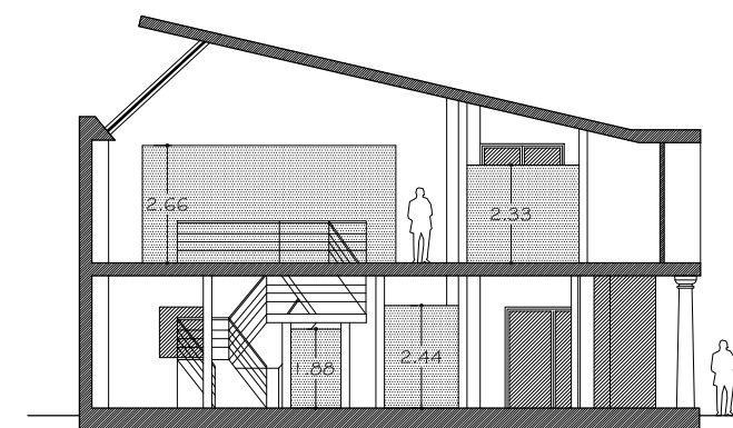
Secció A-A'
