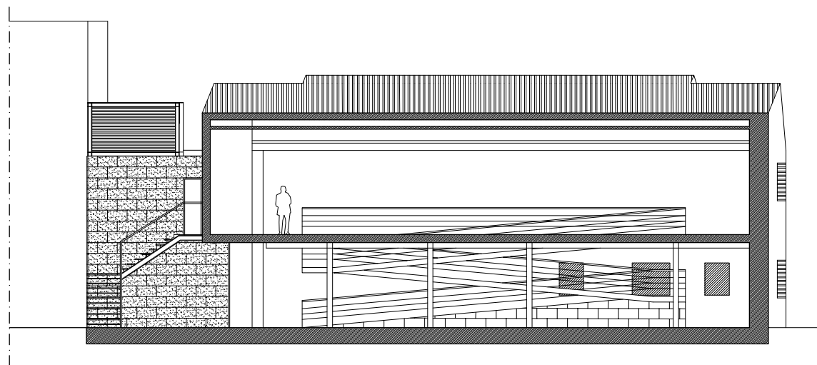
Secció B-B'
